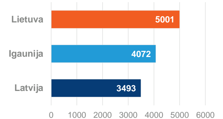
Izmaksas, EUR/km
